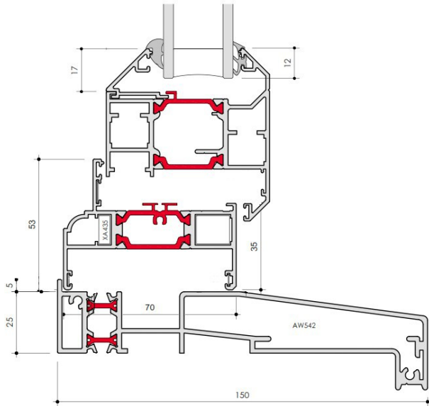
OVOLO (70MM)
