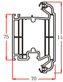
OPEN OUT DOOR SASH P10641
